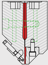
交換式リップ Interchangeable die lip
